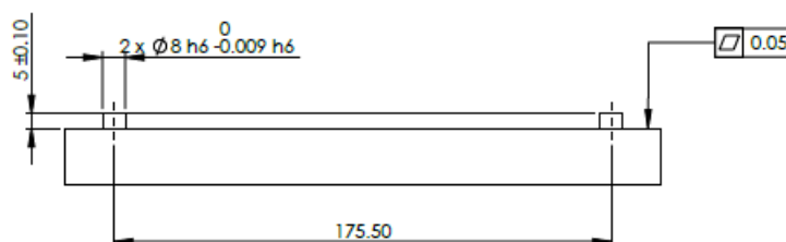
1.2: Montageplaat voor basis van de robot
