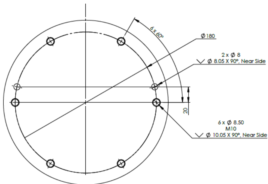
1.1: Onderkant van de basis van de robot
